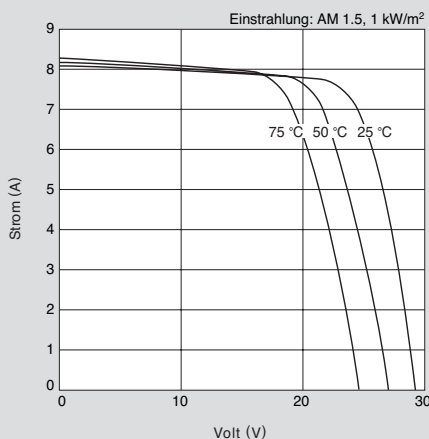
Strom-Spannungs- Kennlinie des Moduls KC175GHT-2 bei verschiedenen Zelltemperaturen.
