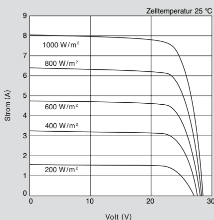
Strom-Spannungs- Kennlinie des Moduls KC175GHT-2 bei verschiedener Einstrahlung.
