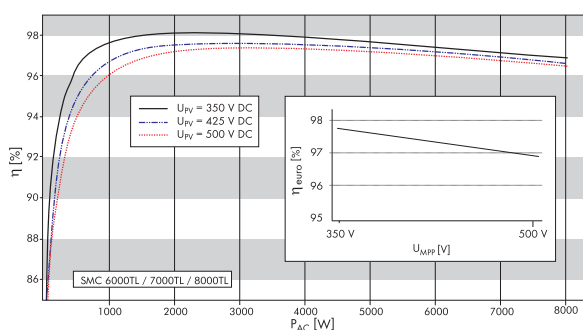
Wirkungsgradkurve
