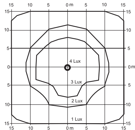
Leuchtcharakteristik aus 4m Lichtpunkthöhe
